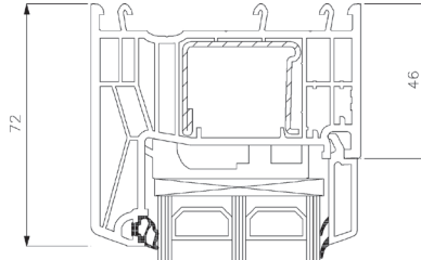
Oberrahmen
