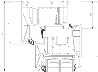
Oberrahmen
