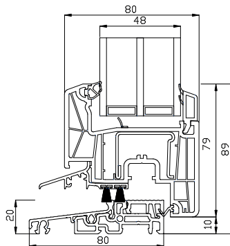
Bodenschwelle Aluminium
