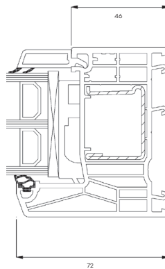
Seitenrahmen
