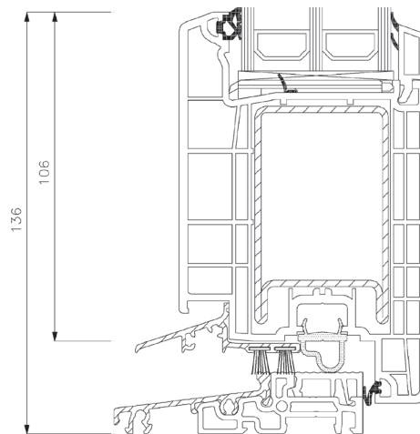
Türschwelle
