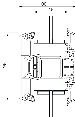
Querprofil
