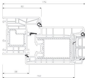
Seitenrahmen
