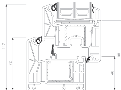
PVC Unterrahmen
