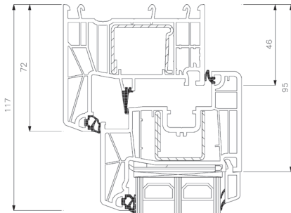
Oberrahmen
