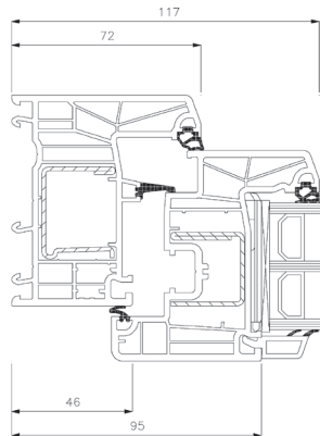
Seitenrahmen
