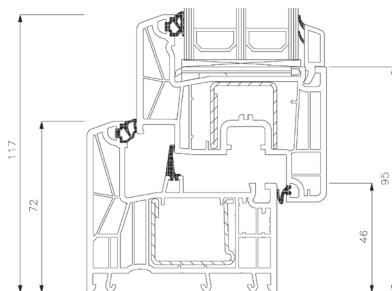
Unterrahmen
