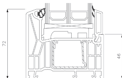
Unterrahmen
