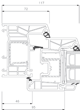
Seitenrahmen
