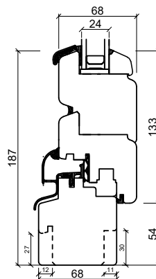
Bodenschwelle Holz
