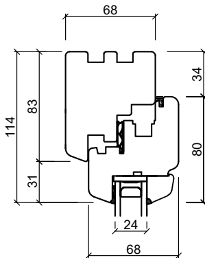
Oberrahmen
