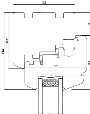
Oberrahmen
