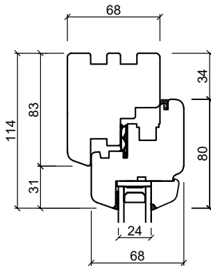
Kämpfer
