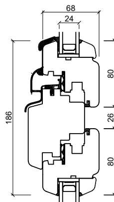
Waagerechter Pfosten
