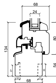
Unterrahmen
