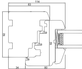
Seitenrahmen
