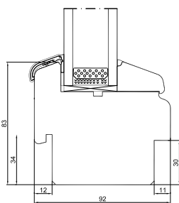
Unterrahmen
