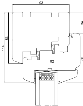
Kämpfer
