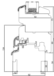
Bodenschwelle Holz
