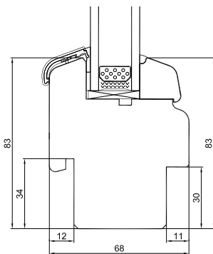
Unterrahmen
