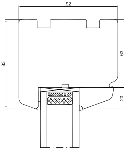
Oberrahmen
