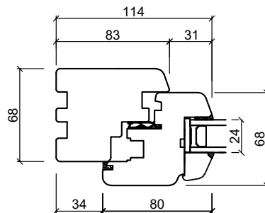
Seitenrahmen
