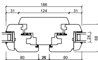
Kämpfer
