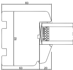
Seitenrahmen
