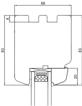
Oberrahmen
