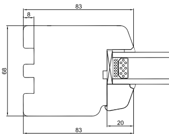
Unterrahmen
