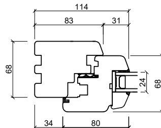
Seitenrahmen
