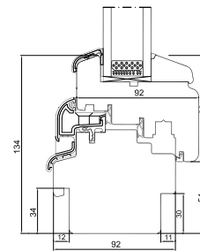
Unterrahmen
