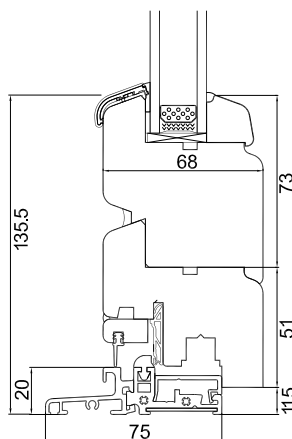
Bodenschwelle Aluminium
