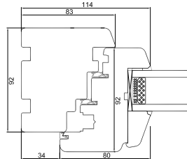
Seitenrahmen
