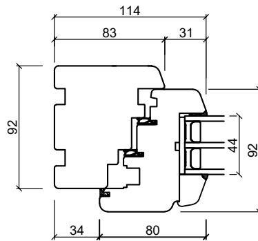
Seitenrahmen
