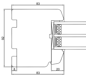
Seitenrahmen
