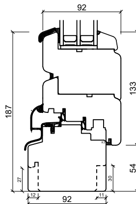
Bodenschwelle Holz
