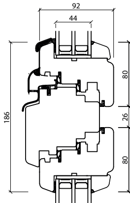
Waagerechter Pfosten
