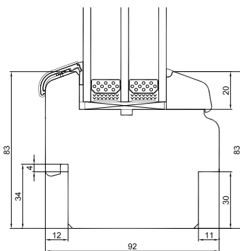
Unterrahmen
