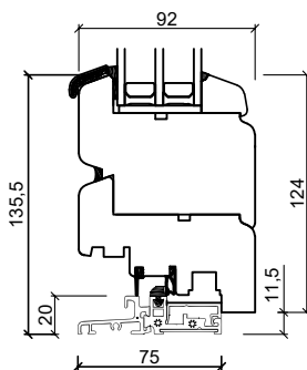
Bodenschwelle Aluminium
