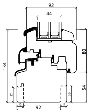
Seitenrahmen
