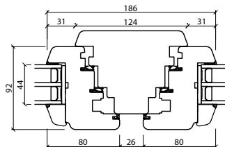
Kämpfer
