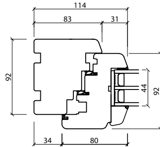
Seitenrahmen
