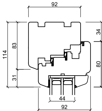
Oberrahmen
