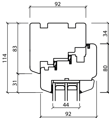
Waagerechter Pfosten
