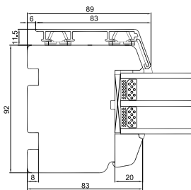
Seitenrahmen
