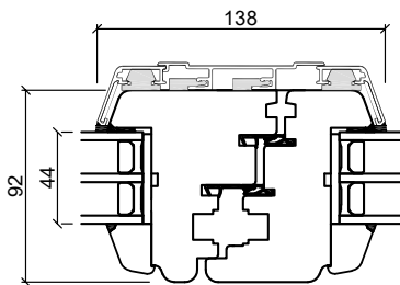
Midt dobbeldør
