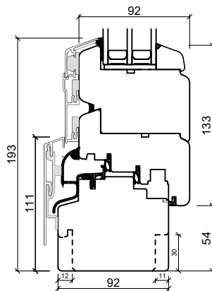
Bodenschwelle Holz
