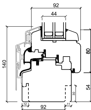
Unterrahmen
