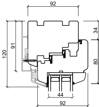
Midt dobbeldør
