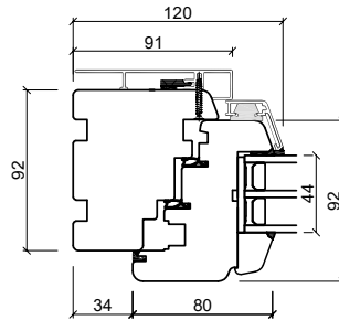
Seitenrahmen
