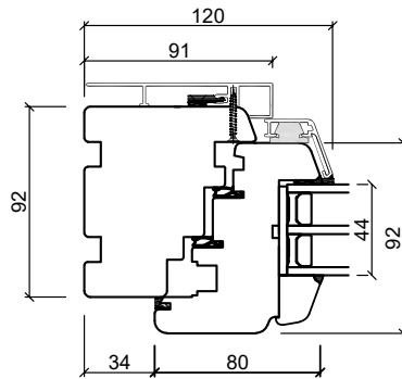
Seitenrahmen
