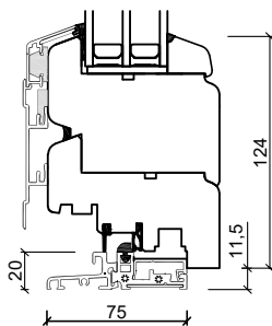
Bodenschwelle Aluminium
