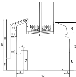
Unterrahmen
