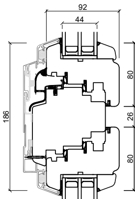
Unterrahmen
