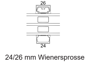
Wienersprosse
