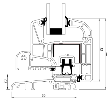
Bodenschwelle Aluminium
