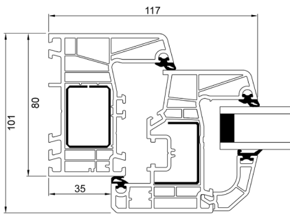
Unterrahmen
