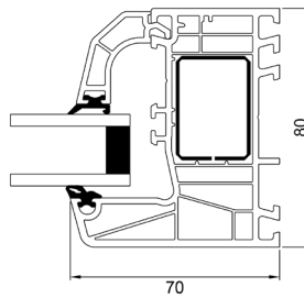
Seitenrahmen
