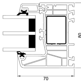
Seitenrahmen
