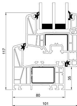
Unterrahmen
