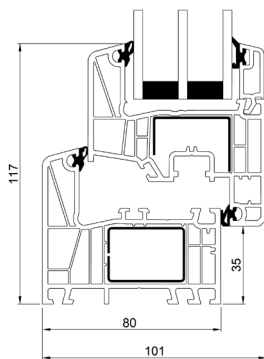
PVC Unterrahmen
