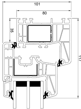
Seitenrahmen
