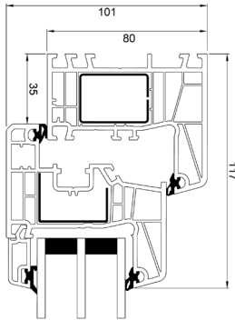
Oberrahmen
