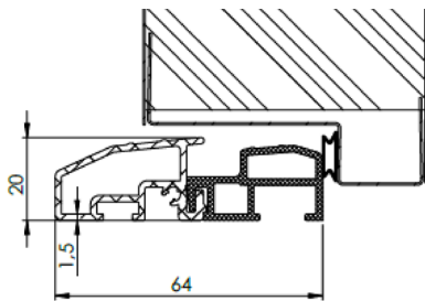
Bodenschwelle Aluminium
