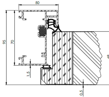
Seitenrahmen
