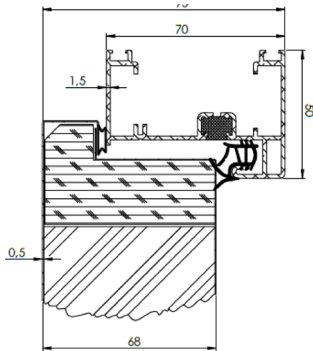
Oberer Türrahmen
