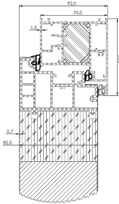
Oberer Türrahmen
