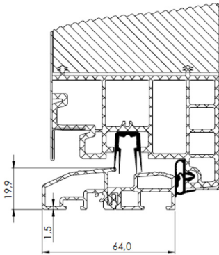
Bodenschwelle Aluminium
