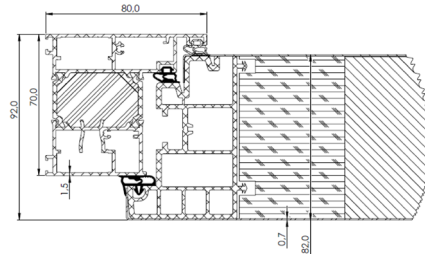
Seitenrahmen
